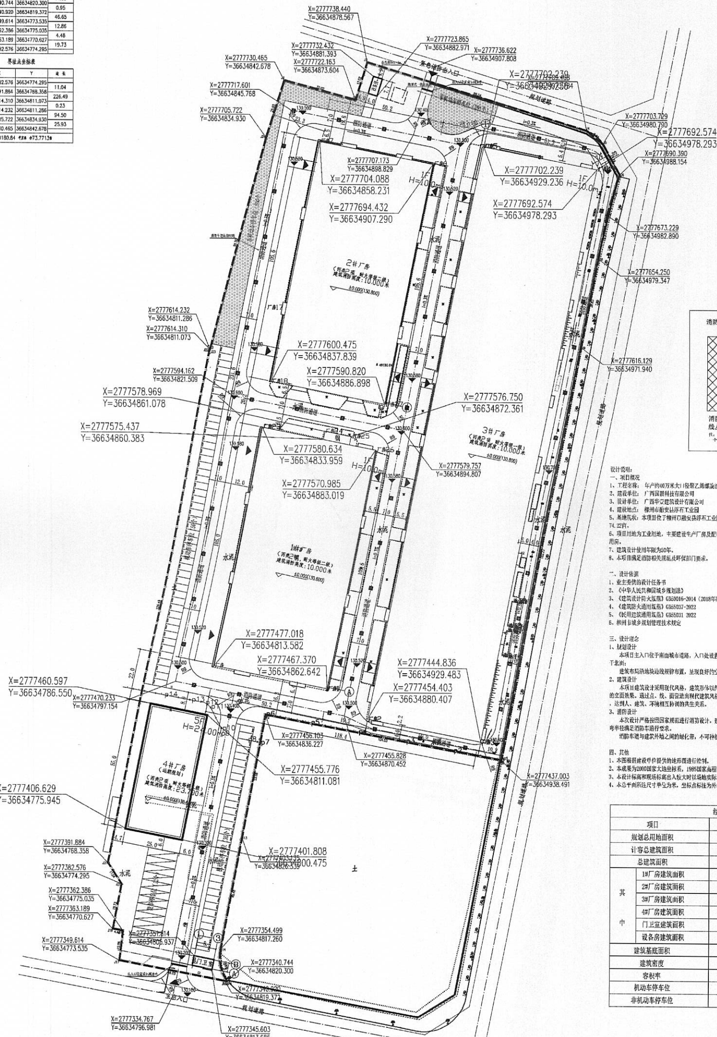
规划总平面图 1:500
