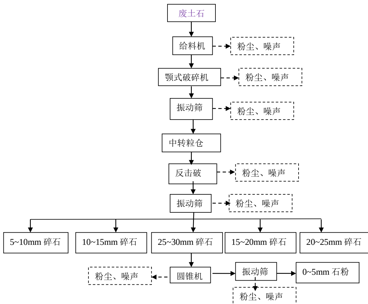
图 5-1 碎石与石粉生产工艺流程图
