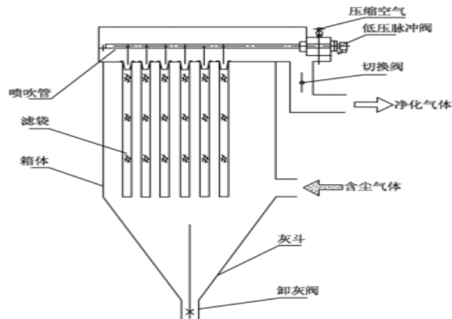
图 7-1 袋式除尘器结构示意图
