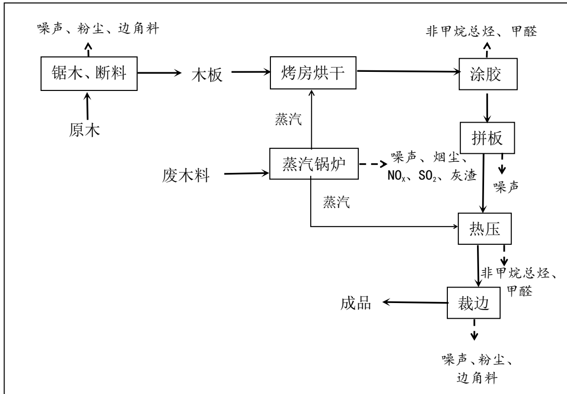
图 1 主要生产工艺流程及产污环节图
