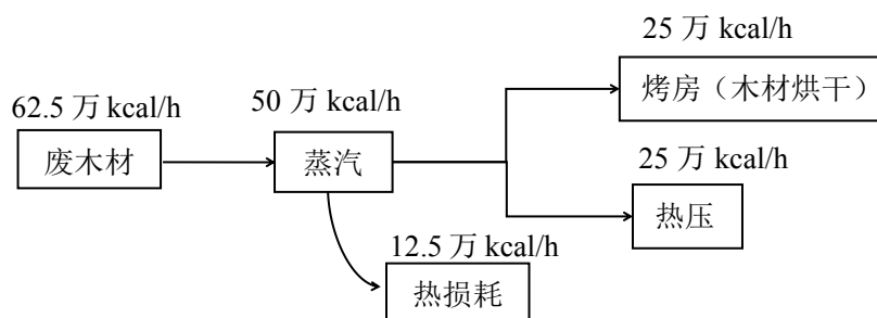
图3 热平衡图
