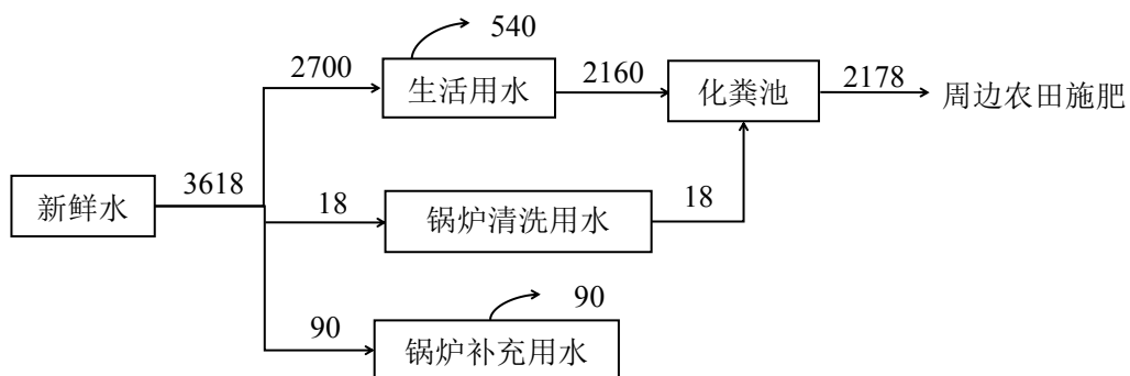
图2 水平衡图 (t/a)
